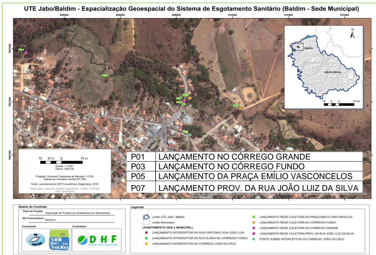
Figura 2.6 – Pontos de lançamento de esgoto in natura , na Sede. Fonte: DHF Consultoria, 2016.
