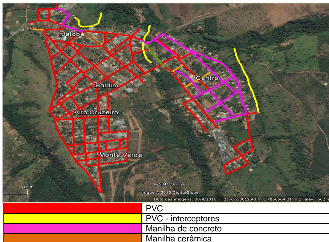
Figura 2.1 – Vista geral da distribuição da rede coletora na Sede municipal de Baldim.
