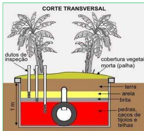
Figura 4.12 – Seção transversal do TEvap.
