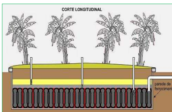
Figura 4.13 – Seção longitudinal do TEvap. Fonte: Kleiton Xavier, 2016.
