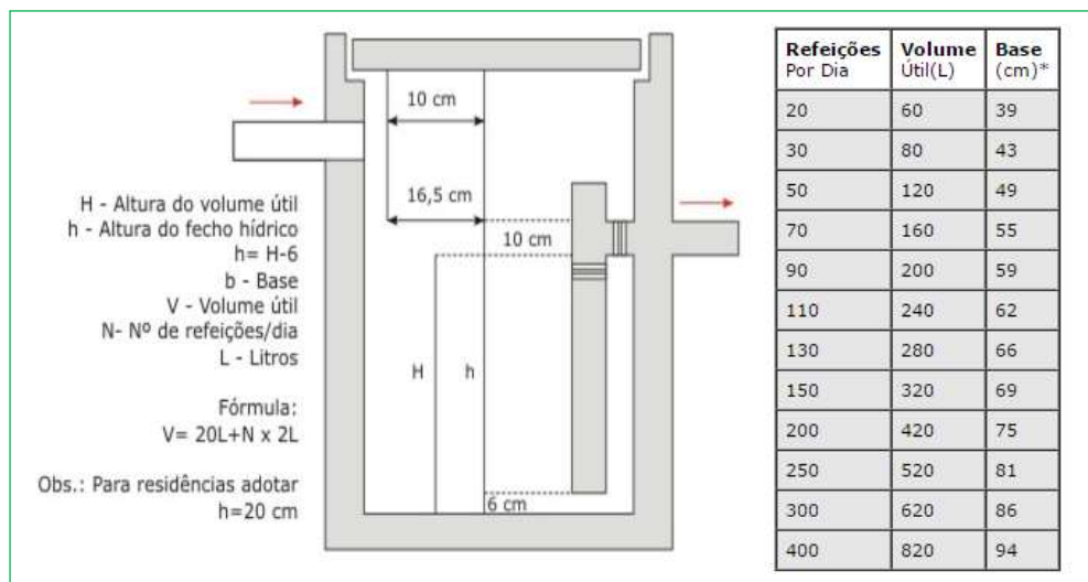
Figura 4.18 – Detalhe Caixa de Gordura e dimensionamento.
