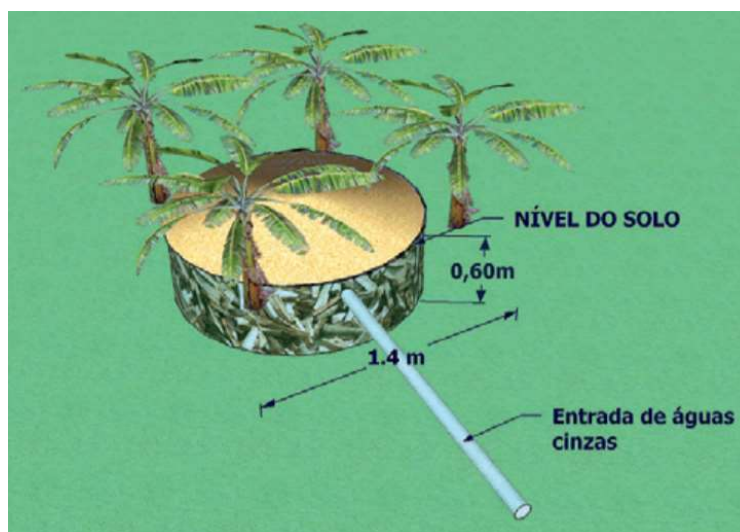
Figura 4.14 – Desenho esquemático do círculo de bananeiras.
