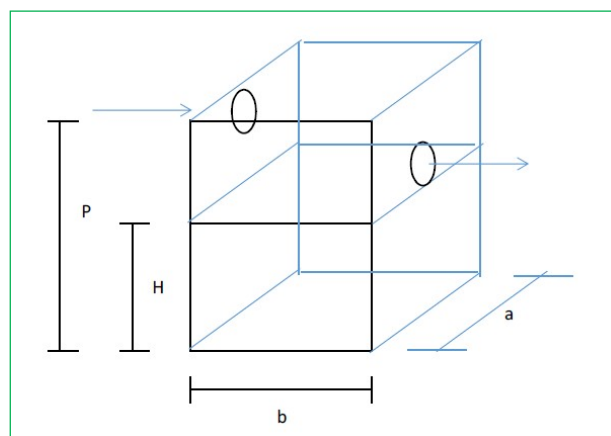
Figura 4.19 - Detalhe dimensões Caixa de Gordura.
