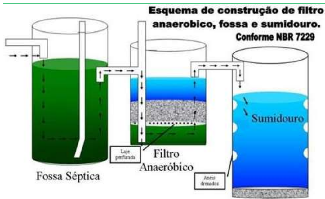
Figura 4.5 – Esquema do conjunto Fossa-filtro-sumidouro.
