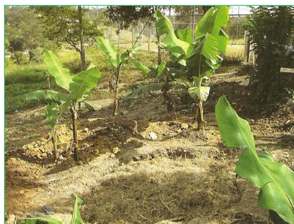
Figura 4.16 – Vala preenchida abaulada e com plantio no entorno Fonte: Leal, 2016.
