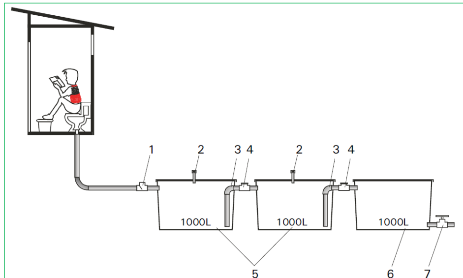
Figura 4.10 – Fossa Séptica Biodigestora para 5 pessoas.
