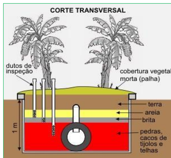
Figura 4.8 – Seção transversal do TEvap. Fonte: Kleiton Xavier, 2016.
