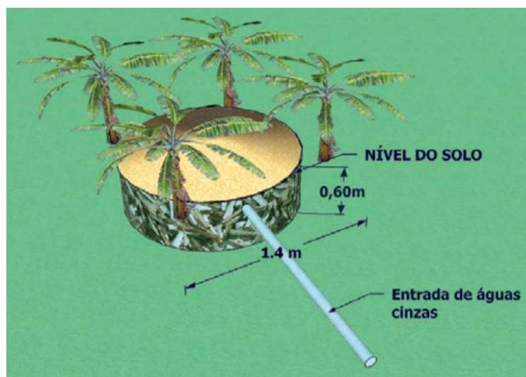
Figura 4.13 – Desenho esquemático do círculo de bananeiras. Fonte: Leal, 2016.
