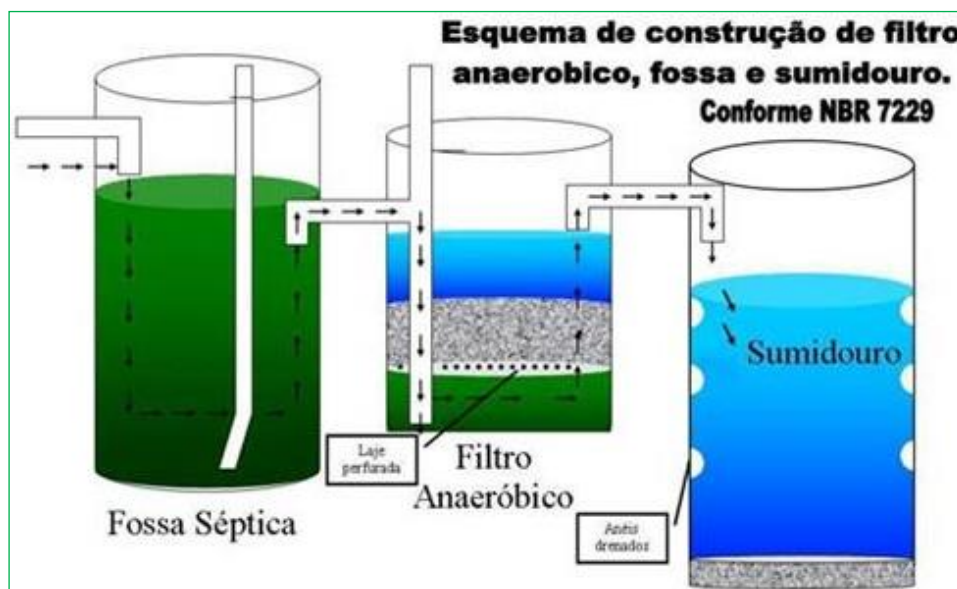
Figura 4.1 – Esquema do conjunto Fossa-filtro-sumidouro. Fonte: MASTER AMBIENTAL, 2016.
