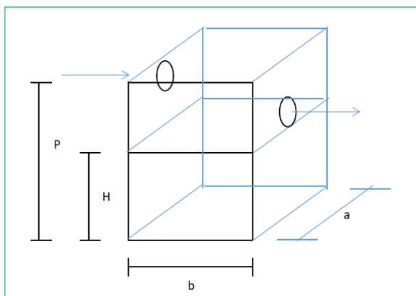
Figura 4.18 - Detalhe dimensões Caixa de Gordura.
