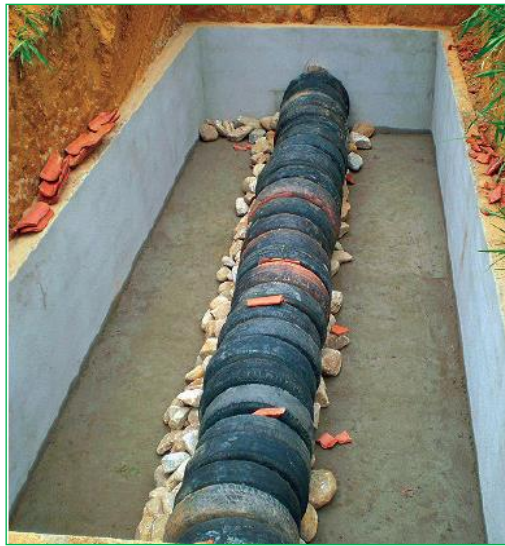
Figura 4.2 – TEvap – Trincheira impermeabilizada e câmara de digestão montada. Fonte: Leal, 2014.
