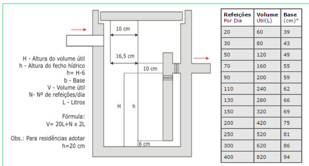
Figura 4.17 – Detalhe Caixa de Gordura e dimensionamento.
