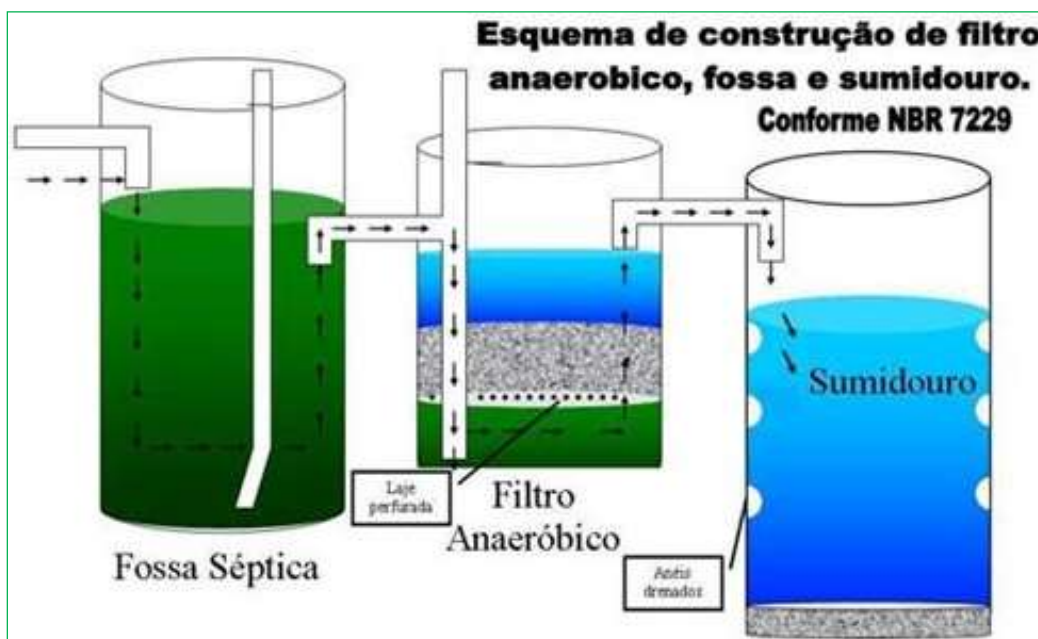
Figura 4.1 – Esquema do conjunto Fossa-filtro-sumidouro. Fonte: MASTER AMBIENTAL, 2016.
