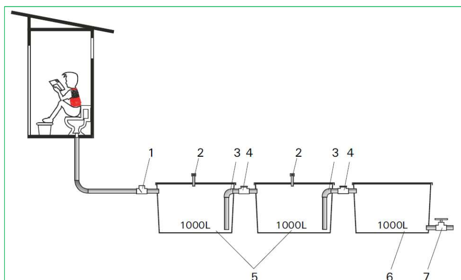
Figura 4.10 – Fossa Séptica Biodigestora para 5 pessoas.
