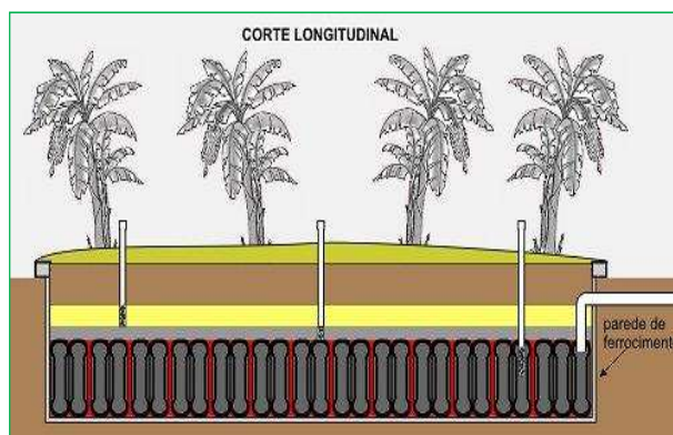
Figura 4.9 – Seção longitudinal do TEvap. Fonte: Kleiton Xavier, 2016.
