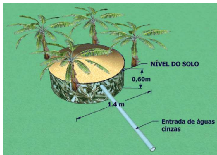
Figura 4.13 – Desenho esquemático do círculo de bananeiras.
