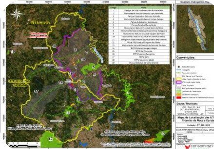
Mapeamento de corredores ecológicos no SAP Vetor Norte – Carste/Ribeirão da Mata
